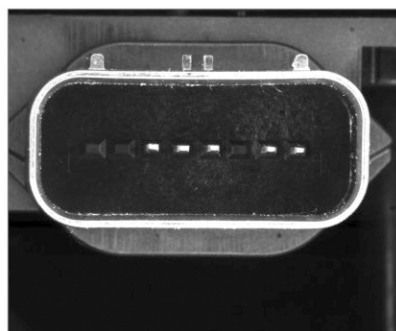
CST-RS10010-W pin脚有无判断
