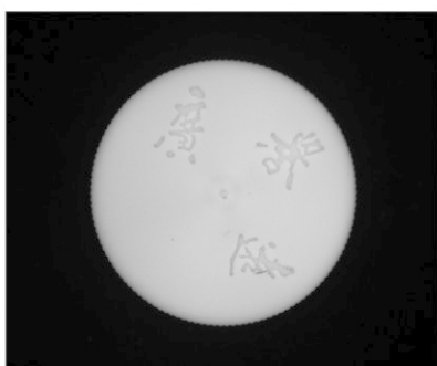
CST-POR8090-W 瓶盖缺陷检测
