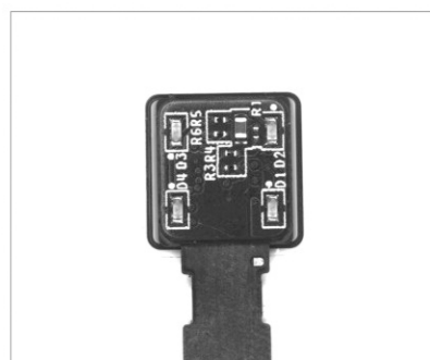
CST-POR8090-W 摄像头模组字符及定位检测
